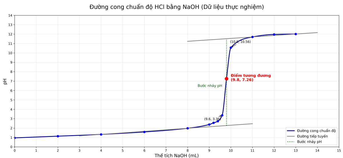
Figure 8.2: Đường cong chuẩn độ HCl 0.1N bằng NaOH 0.1N
